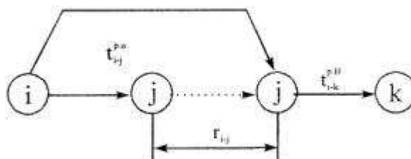
Рисунок 25 - Свободный резерв времени для работы i-j.
