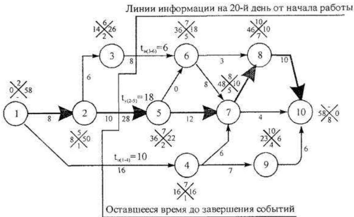
Рисунок 29 - Анализ хода работ по потенциалам событий
