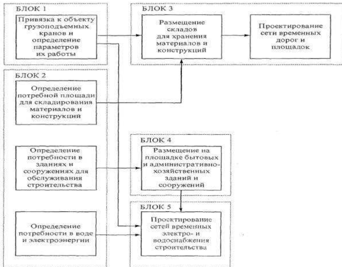
Рисунок 3 - Блок-схема проектирования объектного стройгенплана
