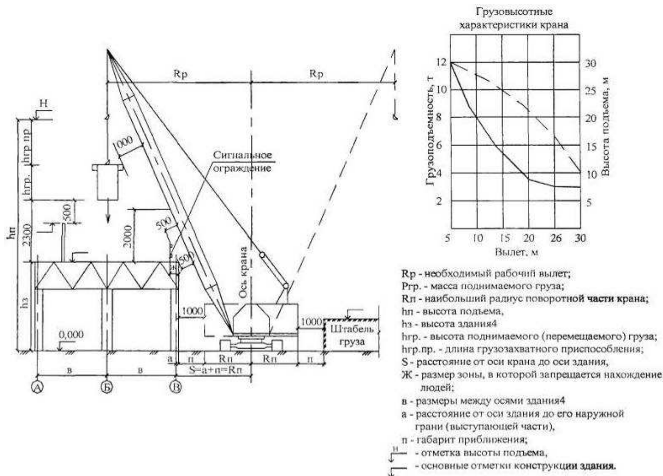
Рисунок 7 - Привязка стрелового крана к зданию
