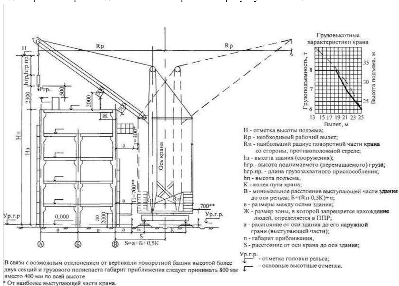
Рисунок 6 - Привязка башенного крана к зданию
