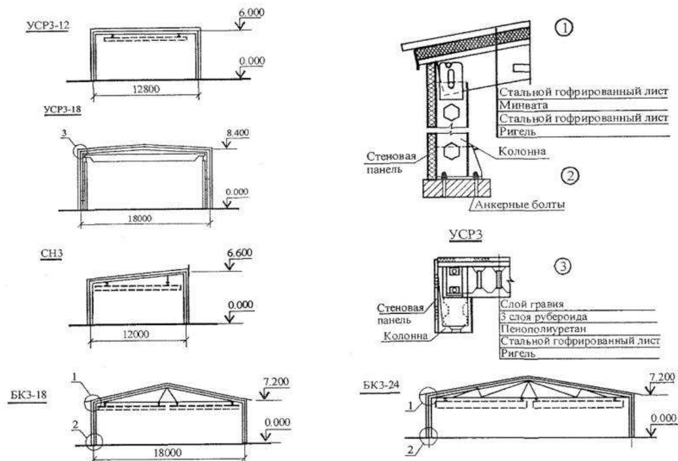
Рисунок 4 - Варианты устройства временных зданий сборно-разборного типа
