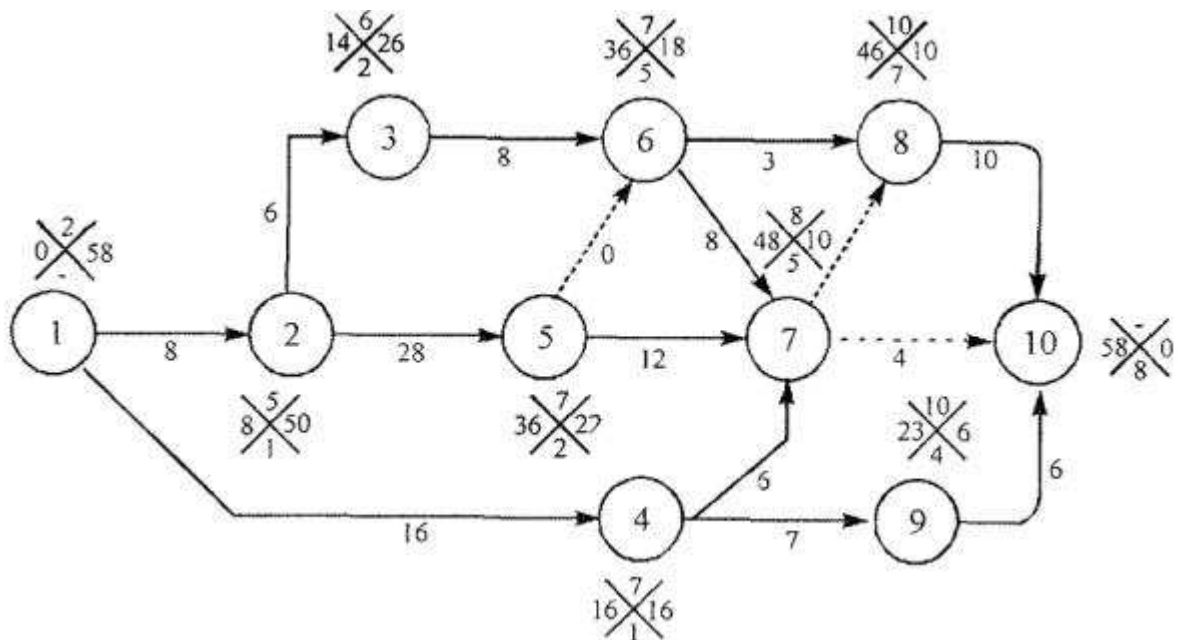
Рисунок 28 - Сетевой график, рассчитанный по потенциалам событий
