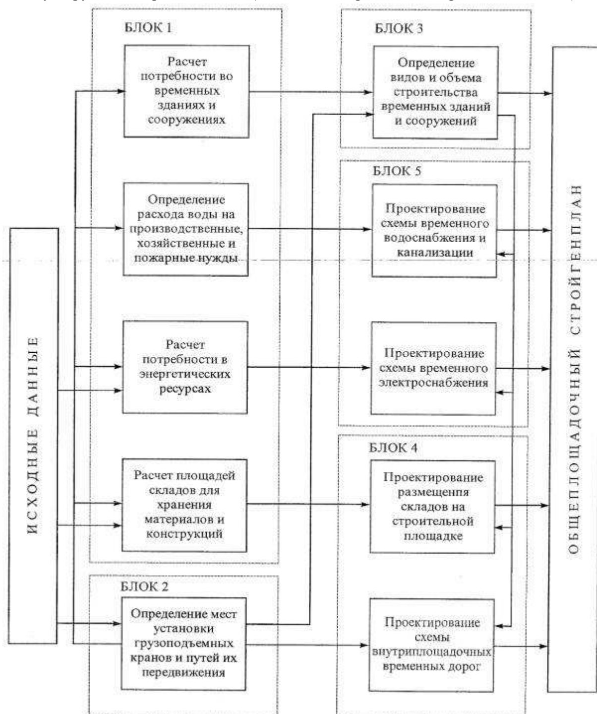
Рисунок 1 - Блок-схема проектирования общеплощадочного стройгенплана
