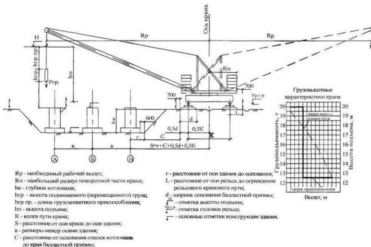
Рисунок 8 - Установка башенного крана у откоса котлована
