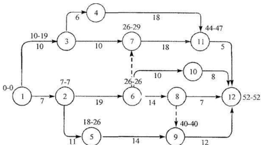
Рисунок 31 - Безмасштабный сетевой график с горизонтальными обозначениями продолжительности выполнения работ
