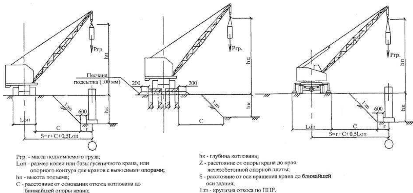
Рисунок 9 - Установка стрелового крана у откосов выемки
