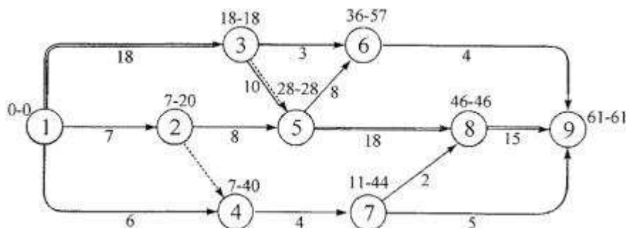
Рисунок 23 - Определение раннего и позднего сроков наступления событий
