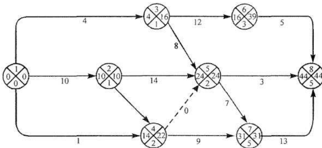
Рисунок 27 - Сетевой график с результатами расчета непосредственно на графике
