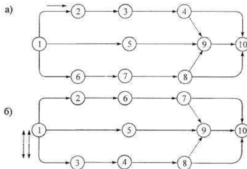
Рисунок 22 - Нумерация событий: а) горизонтальная; б) вертикальная.
