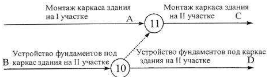
Рисунок 20 - Параллельное выполнение работ А, С и В, Д с фиктивной работой 10-11
