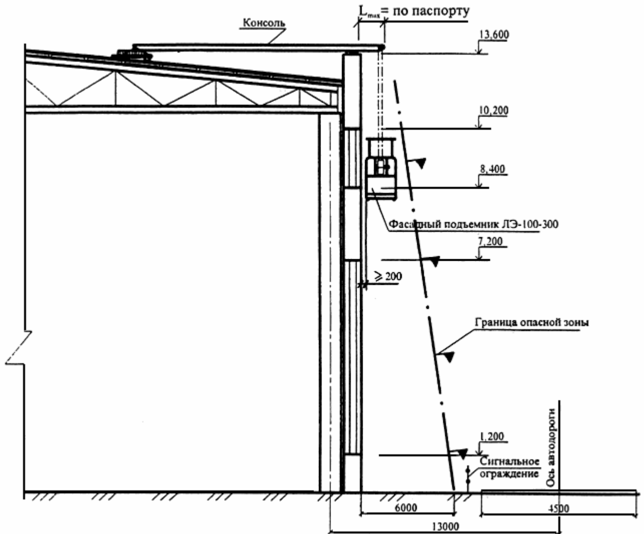
Рисунок 38 - Схема привязки фасадного подъемника для устройства остекления
