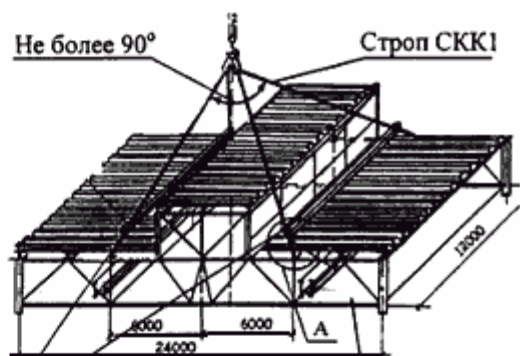
Блок покрытия пром.зданий Р тах =22 т
