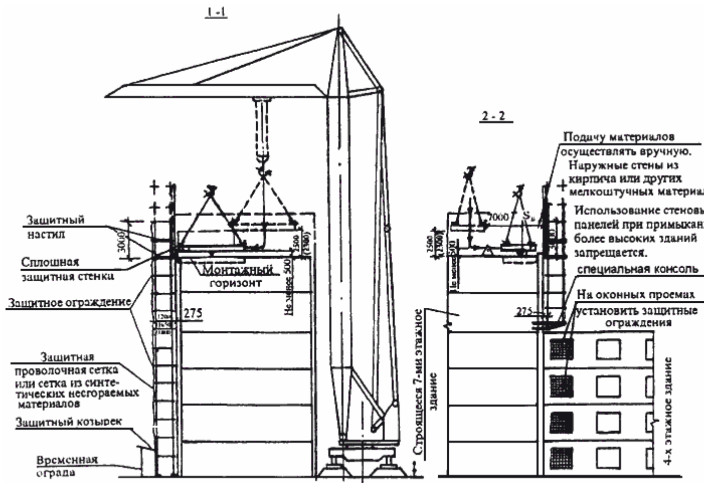
Рисунок 24 - Разрезы 1-1 и 2-2
