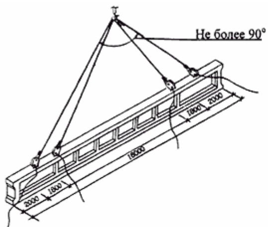
Строп 2СК-10,0
